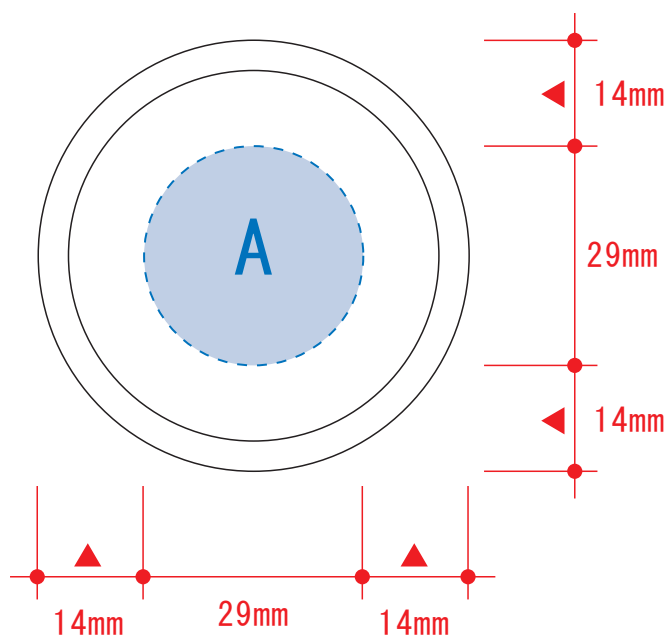
天面 (蓋)
