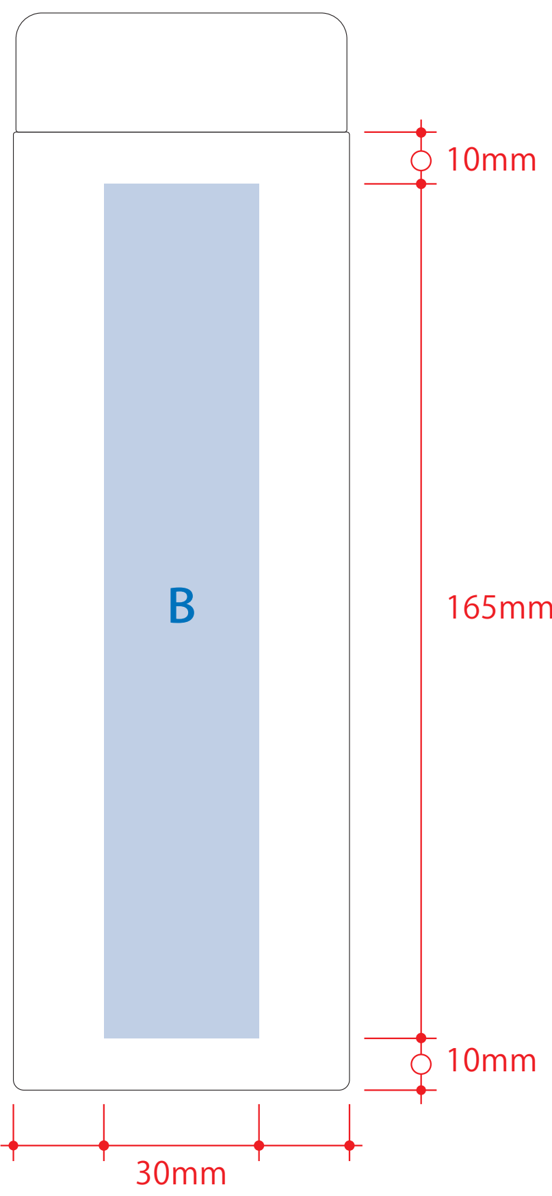
■UV インクジェット印刷 最大範囲： B/W30×H165(mm) C/Φ41 (mm)
